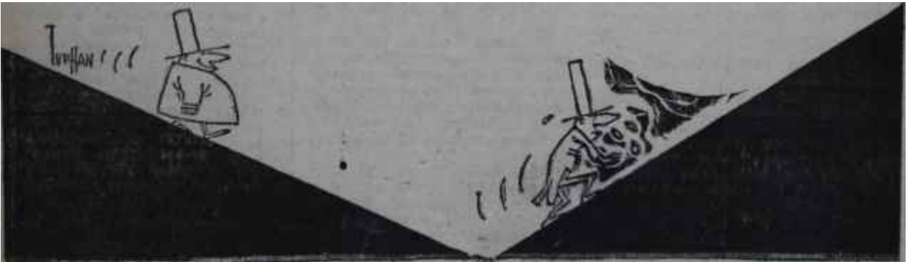
SEÇİM SATHI MAİLİ: İKTİDARA GÖRE
